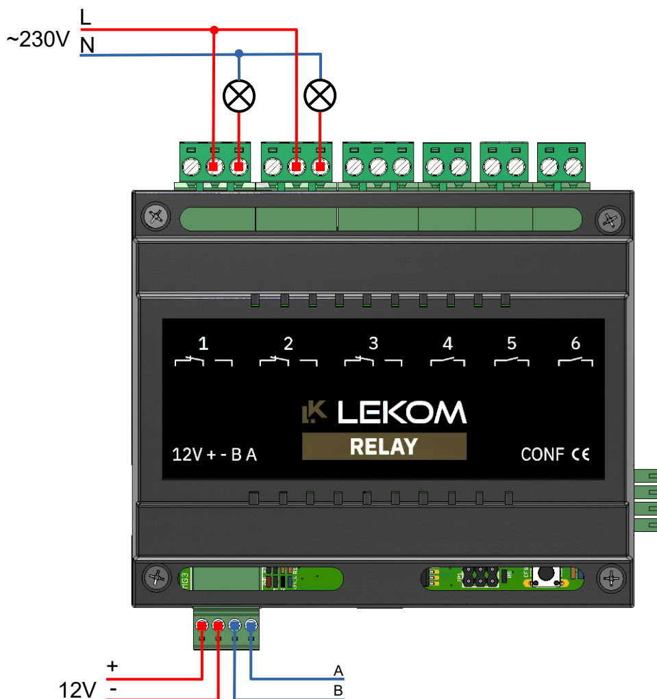
4.3. Przykład podłączenia.
